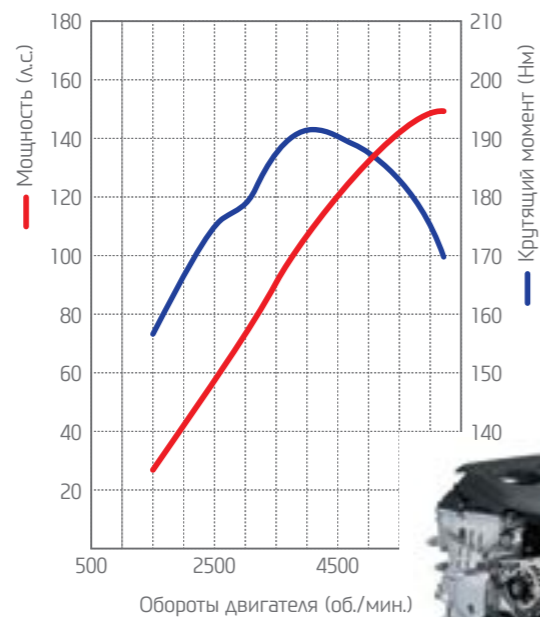
Двигатель Pi 2.0 D-CVVT
