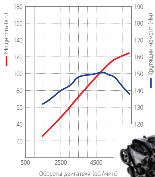
Двигатель Gamma 1.6 D-CVVT
